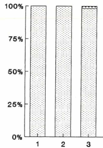
Statusspektren
