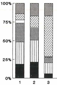
Lebensformenspektren
