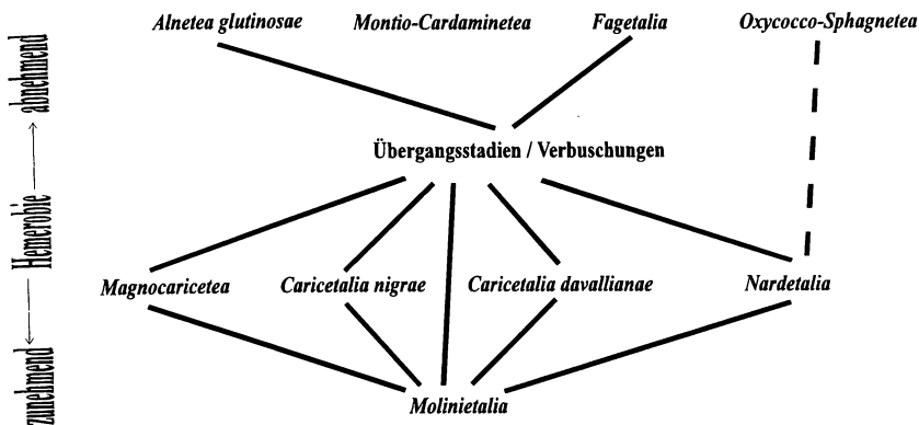
Abb. 3: Entwicklungsbeziehungen der potentiellen natürlichen Vegetation in Abhängigkeit von der Nutzung. Die Y-Achse entspricht dem Grad der Hemerobie. Weitere Erklärungen siehe Diskussion.
