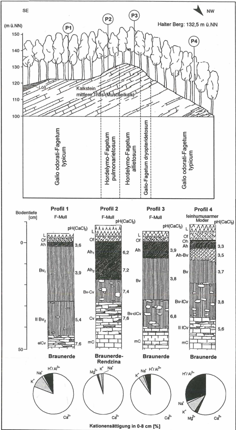
Abb. 2: Vegetationsprofil [oben] und Bodencatena gesellschaftskennzeichnender Humus- und Bodenprofile mit bodenökologischen Charakteristika [unten] anspruchsvollerer Buchenwälder des Galio odorati-Fagenion am Halter Berg im Osnabrücker Berg- und Hügelland (Nordwestliches Weserbergland, Nordwest-Deutschland) (Grundlage HAACK 1930, aus POLLMANN 2000, verändert).
