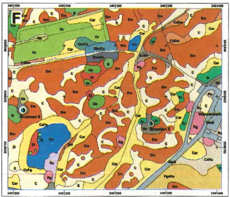
Abb. 27: Datengrundlage und Ergebnisse der Vegetationskartierung am Beispiel eines Detail-Bereiches vom Grundwasser-Einzugsgebiet der Insel Langeoog (A: Deutsche Grundkarte, B: Schwarz-Weiß-Luftbild, C: Color-Infrarot-Luftbild, D: Höhenmodell, E: Feldkarte und F: Vegetationskarte, nach PETERSEN et al. 2003).
