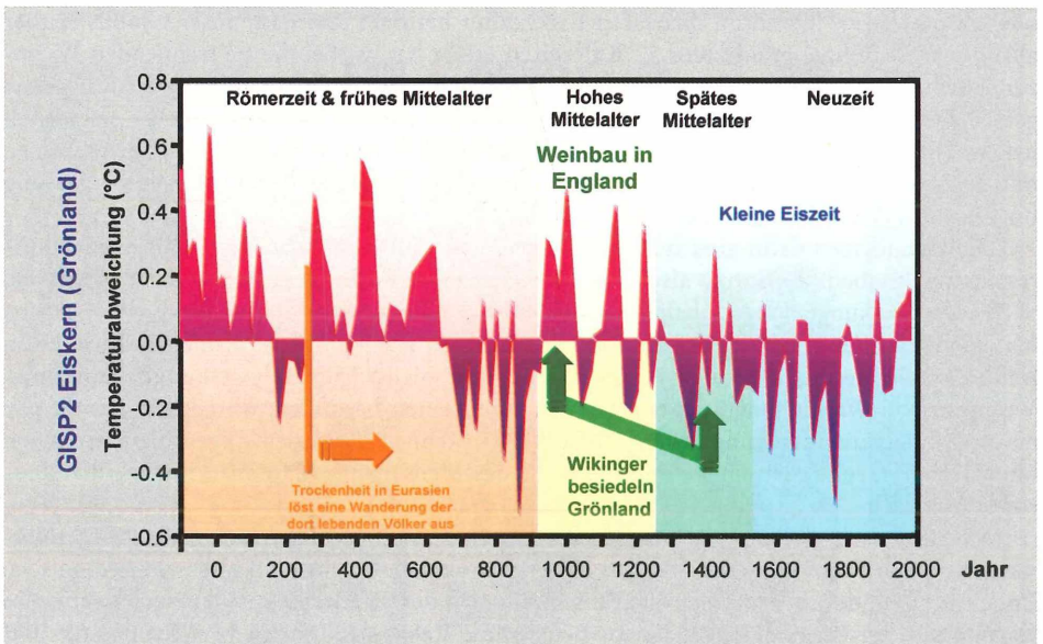
Abb. 22: Paläoökologische Rekonstruktion der Klima- und Landschaftsentwicklung in Mitteleuropa auf der Basis der Korrelation zwischen der rekonstruierten Temperaturkurve aus dem Grönlandeiskern und der Sonnenfleckenaktivität (nach POTT & FREUND 2002).
