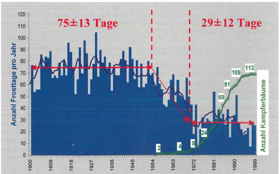
Abb. 19: Temperaturentwicklung und Etablierung von Cinnamomum glanduliferum im Tessin seit 1900 (nach WALTHER 2000, 2002).
