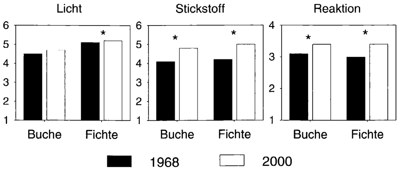
Abb. 4: Mittlere qualitative Zeigerwerte der Kraut- und Moosschicht (Licht und Reaktion) bzw. der Krautschicht (Stickstoff) in Buchen- und Fichtenbeständen im Solling. Vergleich der Aufnahmen von GERLACH (1970) und WECKESSER (2003) aus den Jahren 1966/68 und 1999/2000.
