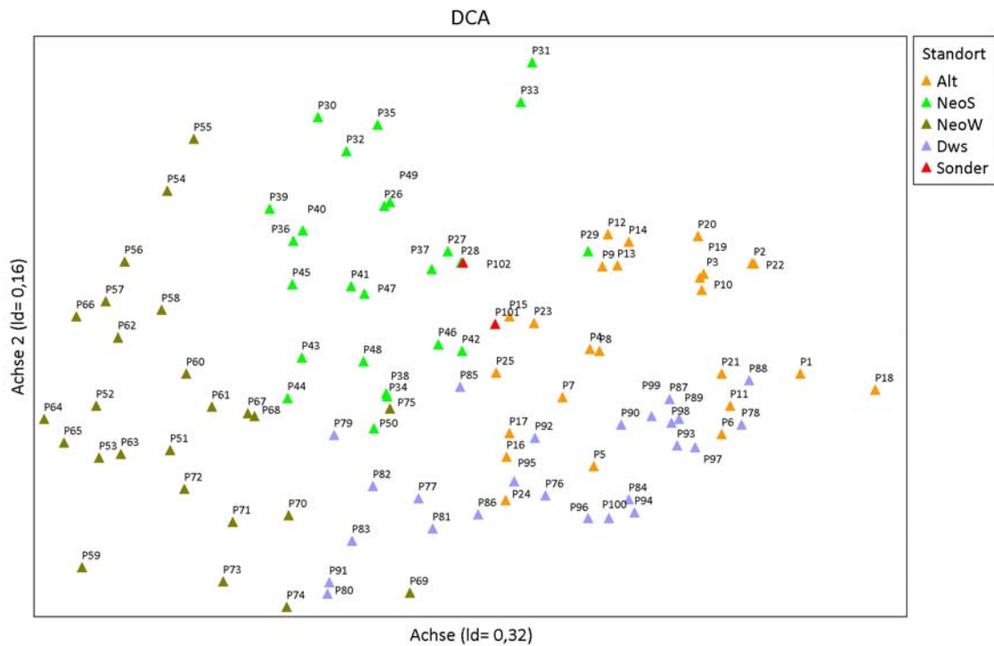
Abb. 2: DCA-Ordinationsdiagramm der pflanzensoziologischen Aufnahmen in den Restitutionsgebieten Hammer und Wester Schleife bei Haselünne (Emsland). 1. und 2. Achse. L_d(\lambda) = Eigenwert der Achsen. Hammer Schleife: SF-HS = Sandfläche in Flussnähe mit spontaner Neubildung, AD-HS = Altdüne mit ursprünglicher Population, WD-HS = „Neodüne“ im Westen, SD-HS = „Neodüne“ im Süden; Wester Schleife: D-WS = „Neodüne“.
